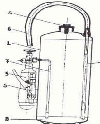
Πυροσβεστήρας ξηρ
