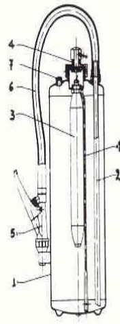
Πυροσβεστήρες ξηράς σκόνης με εσωτερικό φιαλίδιο
